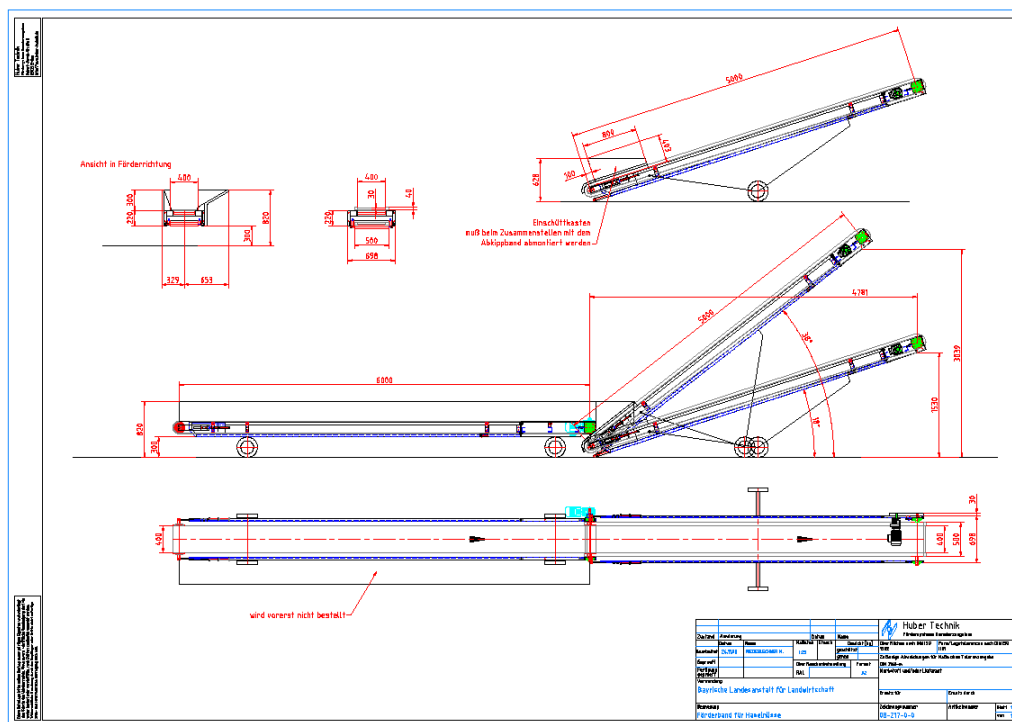
Abbildung 23: Konstruktionszeichnung Förderband
