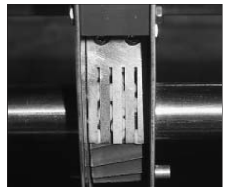
Bild 1: Dosierorgan (Zellenrad) mit Abstreifer
