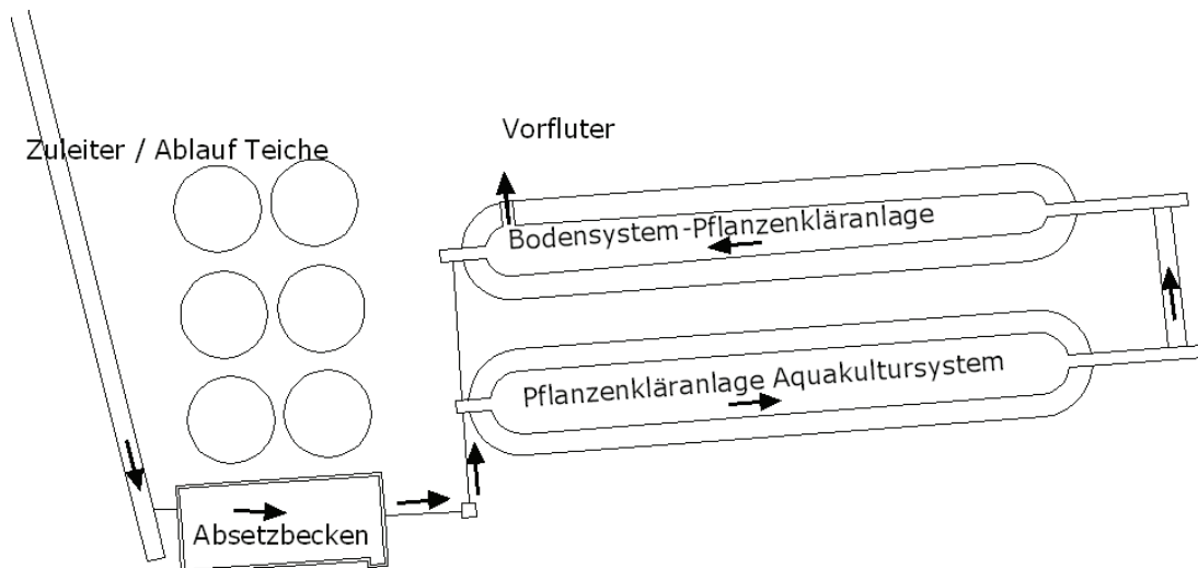
Abb. 12: PKA der Forellenzucht Juraquell, Lageplan
