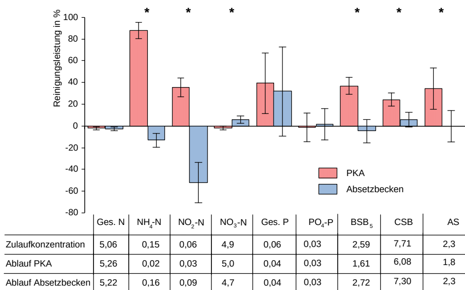
Abb. 14: Reinigungsleistung [%] der PKA am IFI im Vergleich zu Absetzbecken, bei Reinigung des Durchlaufwassers (identische Nährstoffbelastung des Zulaufwassers, * gibt signifikante Unterschiede an, Tabellen-Angaben in mg/L)
