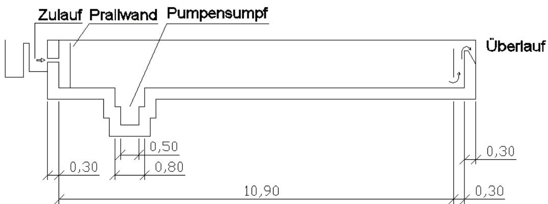
Abb. 10: Schnitt durch ein bestehendes Absetzbecken am IFI (Angaben in Meter)
