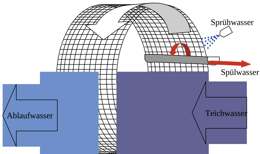
Abb. 19: Funktionsskizze eines Mikrosiebes (blaue Pfeile: Fließrichtung des Wassers, rote Pfeile: auf der Filtergaze zurückgehaltene und abespülte Partikel)
