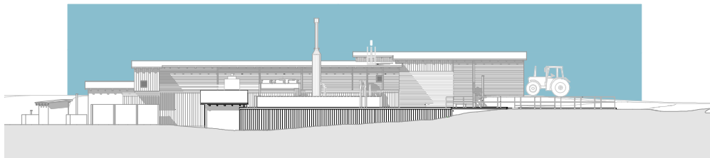
Ansicht Süden
