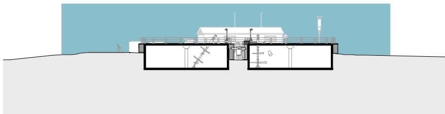
Schnitt A-A
