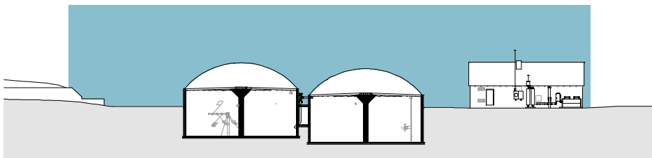
Schnitt
