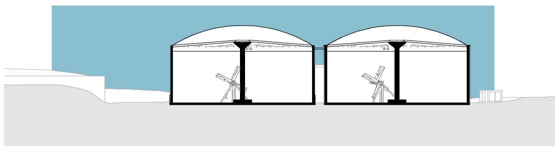
Schnitt A-A
