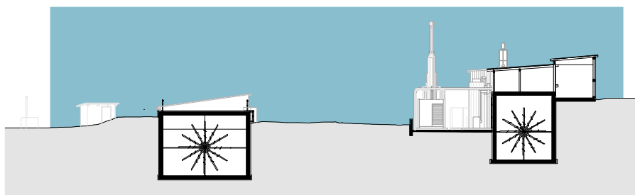
Schnitt A-A
