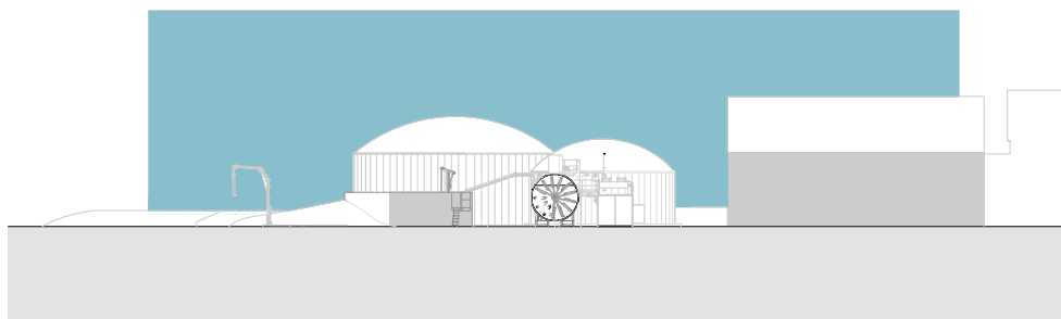
Schnitt A-A
