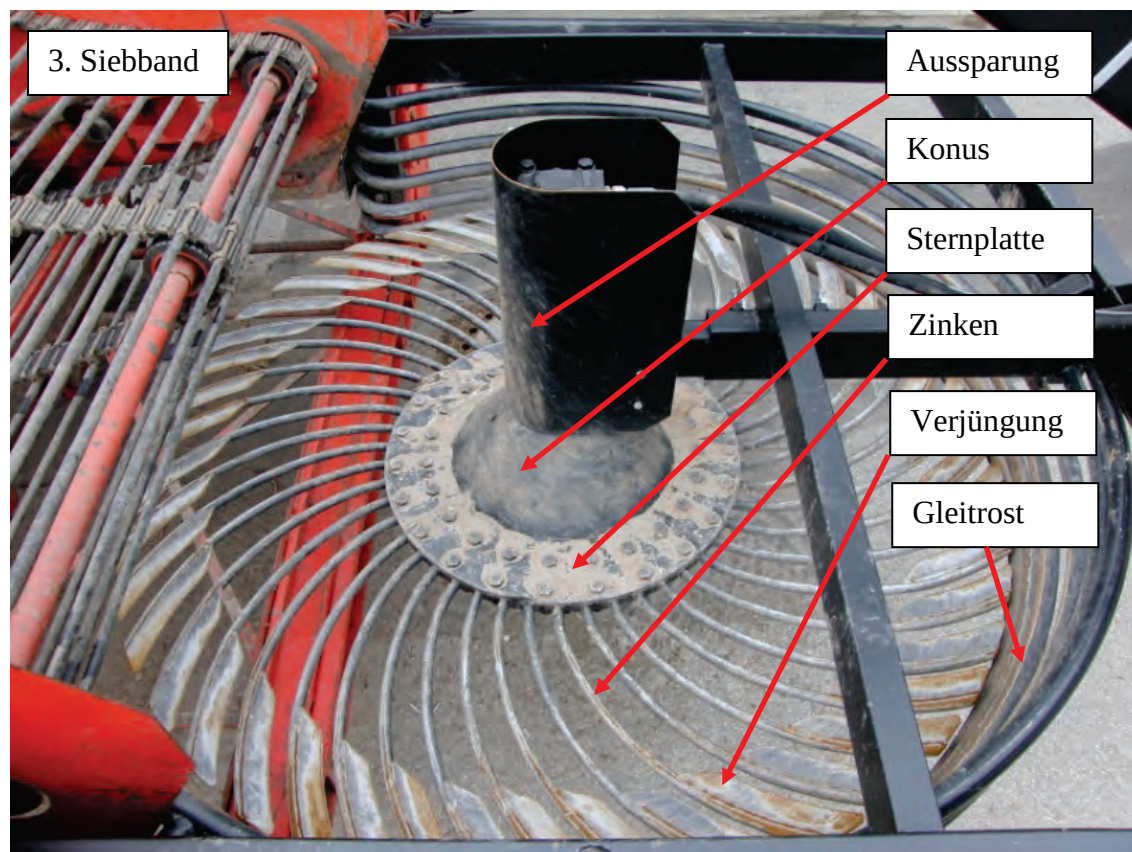
Abb. 37: Siebstern mit Ölantrieb
