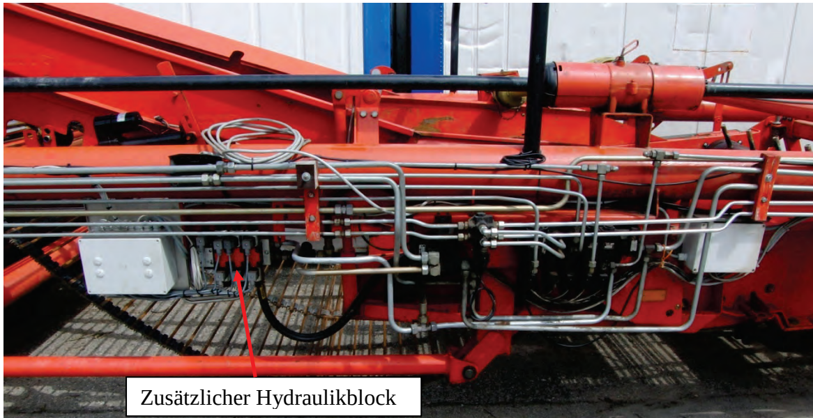
Abb. 47: Hydrauliksteuerventile
