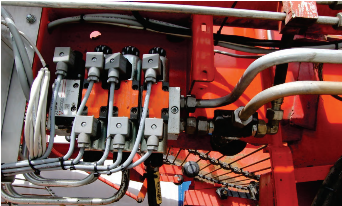
Abb. 48: Zusätzlicher Hydraulikblock mit vorgeschaltetem Mengenteiler
