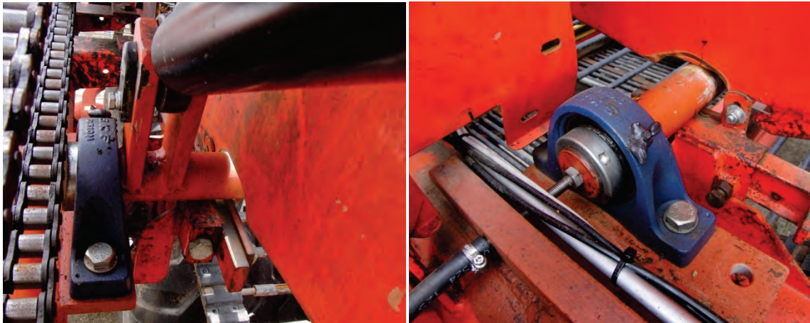
Abb. 30: Lagerung (links) linksseitig, (rechts) rechtsseitig von der Verstellachse im 3. Siebband
