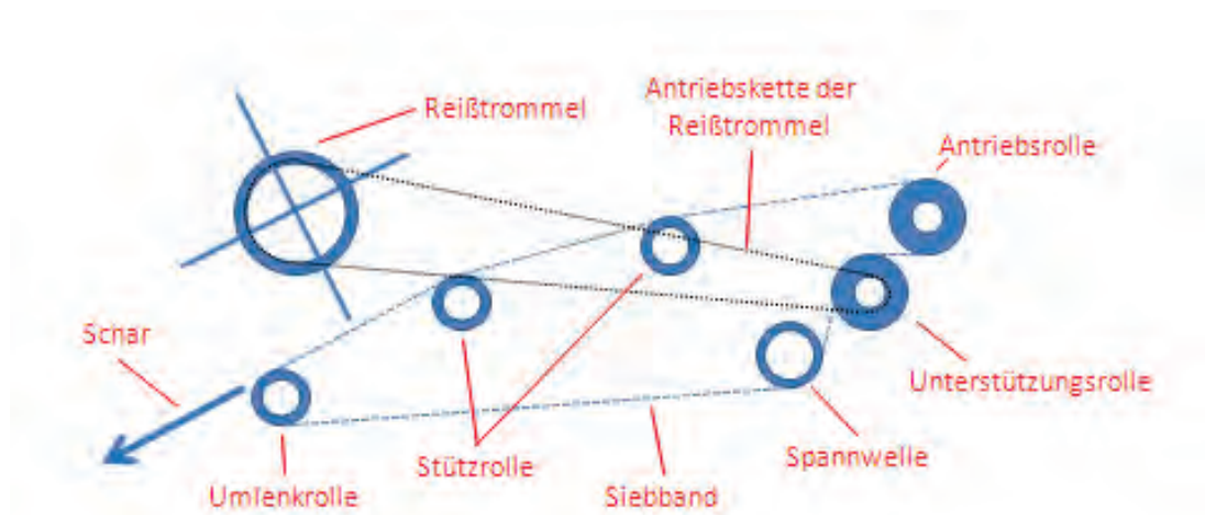
Abb. 6: Skizze zur Positionierung der Reißtrommel
