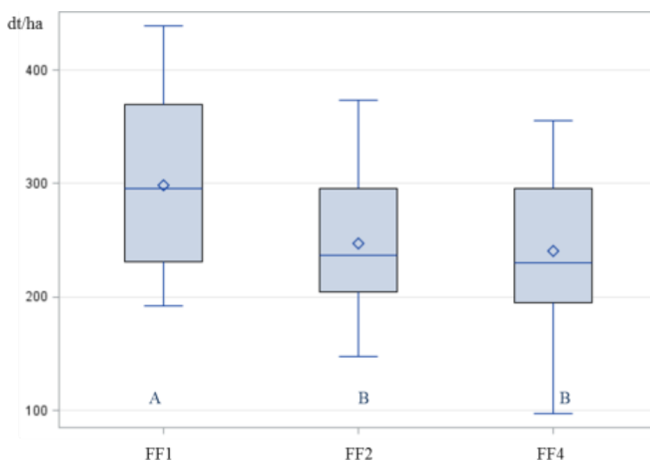
Abb. 29: Mittlerer Knollenertrag in Puch. Unterschiedliche Buchstaben = signifikante Unterschiede ( p \leq 0,05 ) nach dem Student-Newman-Keuls Mittelwerttest.
