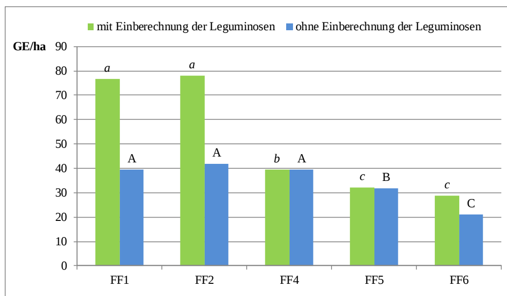
Abb. 40: Durchschnittliche jährlich erzielte Getreideeinheiten pro Hektar und Fruchtfolge in Puch mit und ohne Berücksichtigung der Leguminosen. Unterschiedliche Buchstaben = signifikante Unterschiede ( p \leq 0,05 ) nach dem Student-Newman-Keuls Mittelwerttest.
