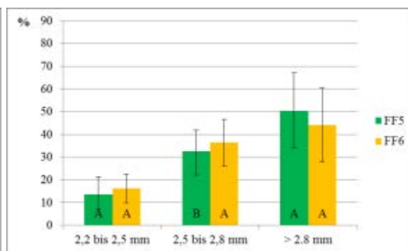
Abb. 20: Sortierung der Sommergerste in Viehhausen. Unterschiedliche Buchstaben = signifikante Unterschiede nach SNK-Mittelwerttest ( p \leq 0,05 )
