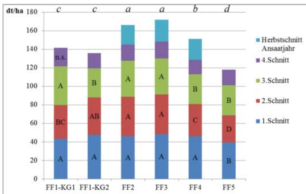
Abb. 8: Mittlere Trockenmasseerträge (2005-2013) der vier Schnitte im Hauptnutzungsjahr und der teilweise durchgeführten Schnitte im Herbst von Klee gras in Viehhausen. Unterschiedliche Buchstaben = signifikante Unterschiede ( p \leq 0,05 ) nach dem Student-Newman-Keuls Mittelwerttest. Buchstaben oberhalb der Säulen beziehen sich auf die Summe Trockenmasse aller Schnitte
