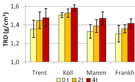
Abb. 1: Trockenrohdichte im Jahr 2009 der vier Versuche ohne Belastung (0 t), mit 2 t und 4 t Radlast
