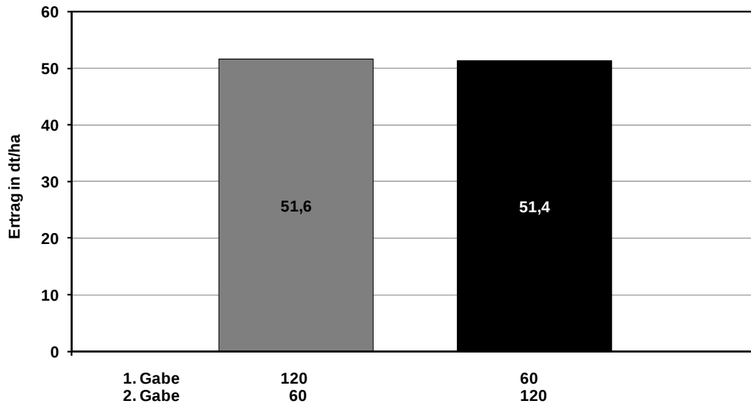
Abb. 3: N-Düngeverteilung im Frühjahr, Mittel aller Orte und Jahre; n=10
