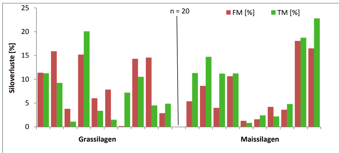
Siloverluste in Frischmasse (FM) und Trockenmasse (TM) bei Gras- und Maissilagen der LVFZ
