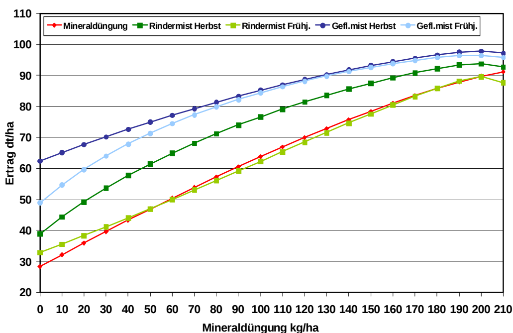
Vergleich der N-Ertragskurven verschiedener Stallmistarten nach Boguslawski/Schneider, Winterweizen 2006
