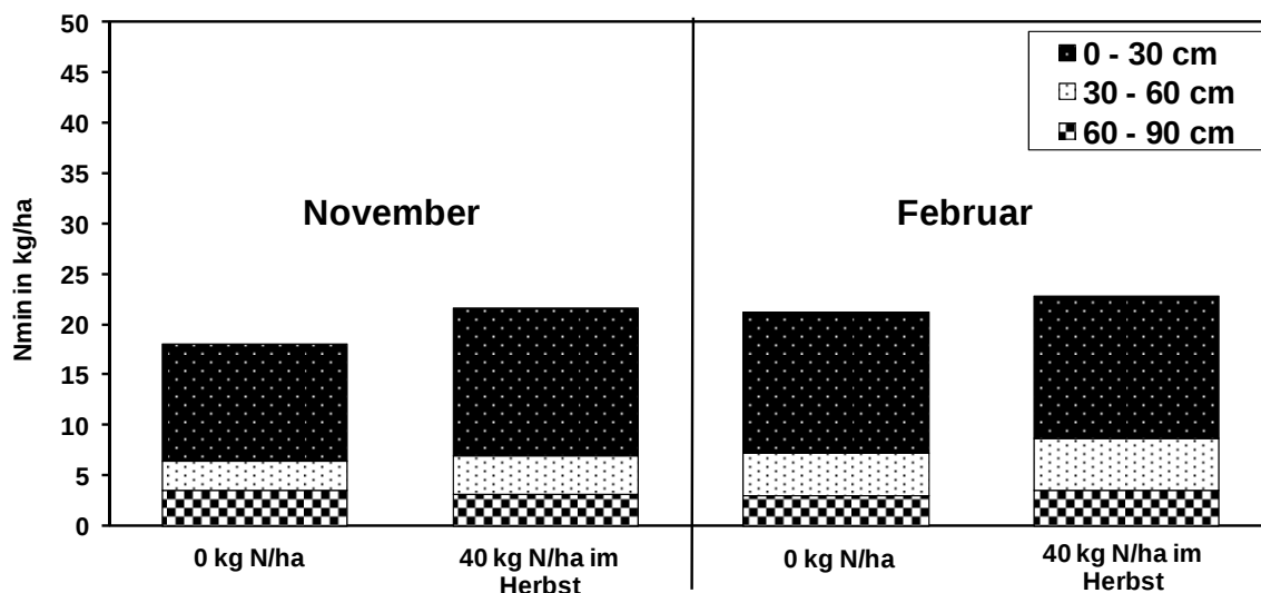
Abb. 2: N_{\min} -Gehalt in Abhängigkeit von einer Herbsdüngung, Mittel aller Orte, Jahre 2008 bis 2010 (Rapssaat bis Ende August)
