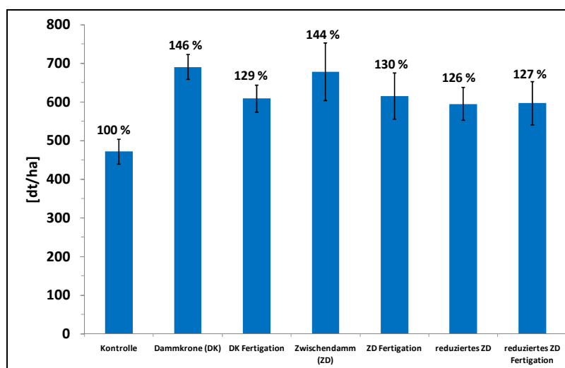
Erträge am Versuchsstandort Abenberg in Abhängigkeit der Tropfschlauchposition und der Düngung
