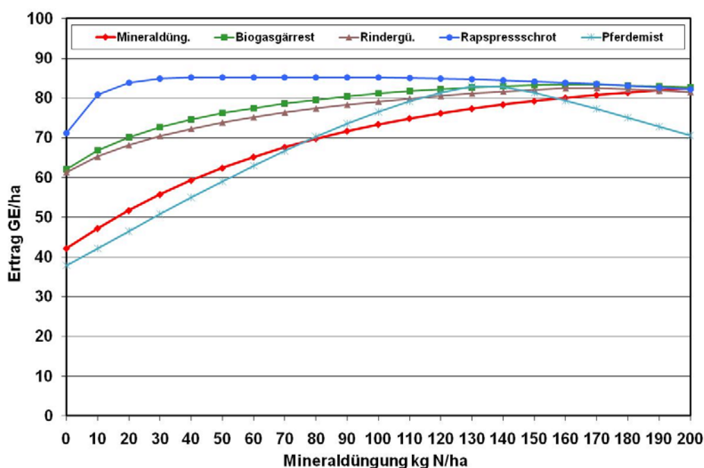
N-Ertragskurven der verschiedenen organischen Dünger (nach Boguslawski/Schneider), Ertragsmittel aus 2007 bis 2009
