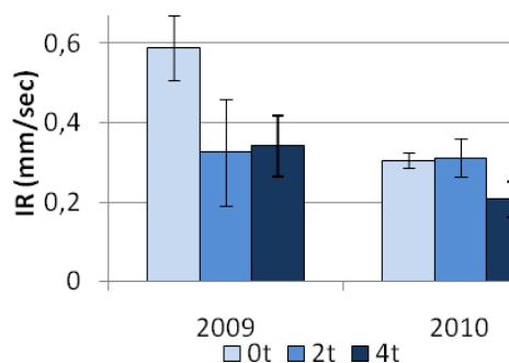
Abb. 2: Infiltrationsrate in Mammendorf ohne Belastung (0 t), mit 2 t und 4 t Radlast in den Jahren 2009 und 2010
