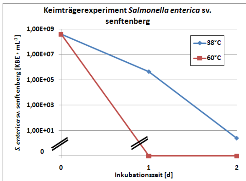
Keimreduktion von Salmonellen im Biogasprozess bei 38°C und 60°C
