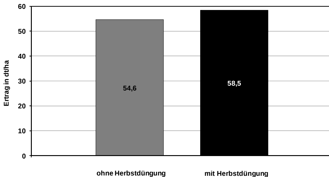
Abb. 1: Winterrapsertrag in Abhängigkeit von einer Herbstdüngung, Mittel von Oberhummel, Jahre 2008 bis 2010
