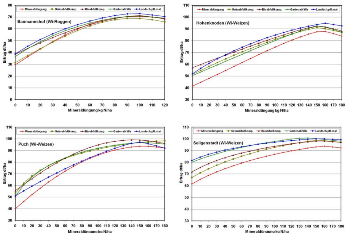
N-Ertragskurven nach Boguslawski/Schneider
